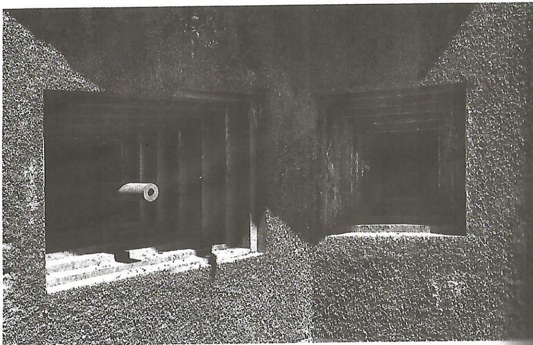
Créneaux de tir de l'entrée des munitions. Dans le créneau de gauche, un canon antichar de 47 mm.
