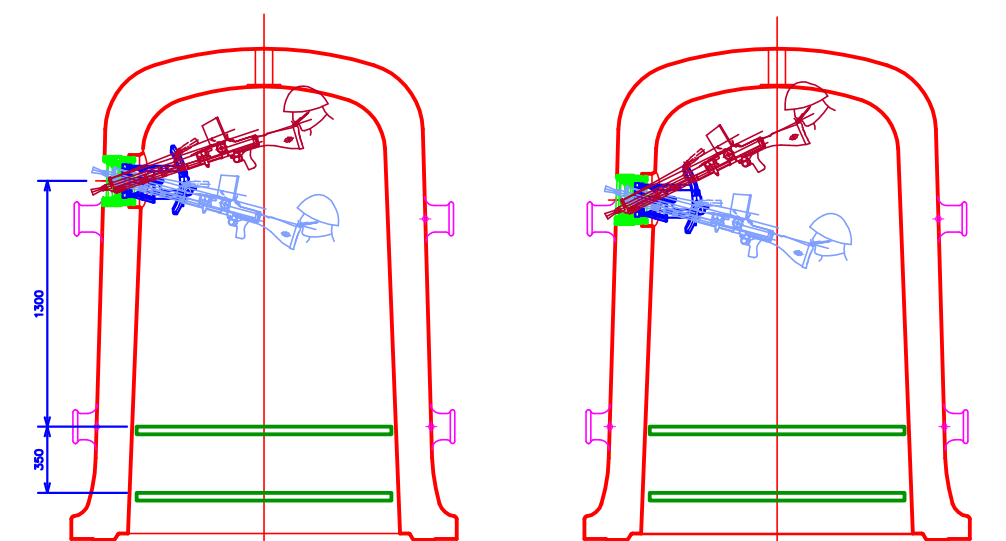
Pointage vertical pour 15°/1:3
