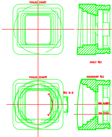
Créneau – cadre fixe pour élévation 15° et dépression 1:2
