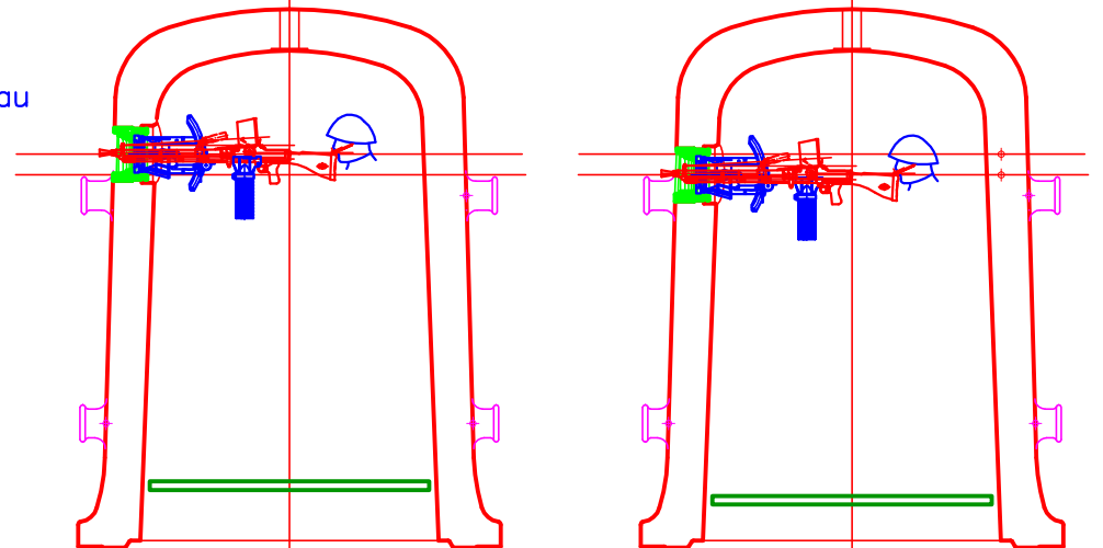
Installation de FM pour dépression 1:2
