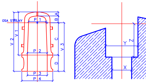
Dimensions générales pour placement
