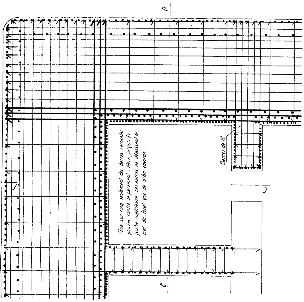
Fig 3. Plan partiel d'une couche de barres. Coupe suiv' AB
